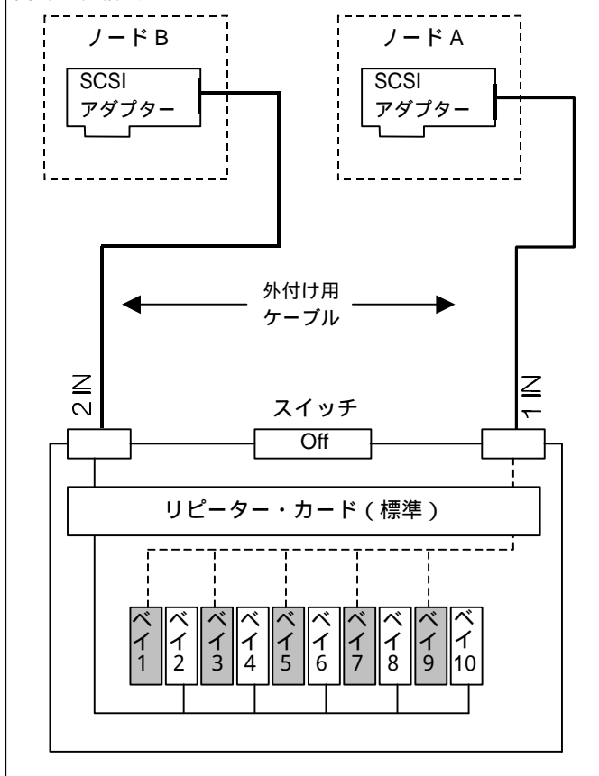
EXP200 を 1 つの SCSI バスに接続する場合 高可用性構成
