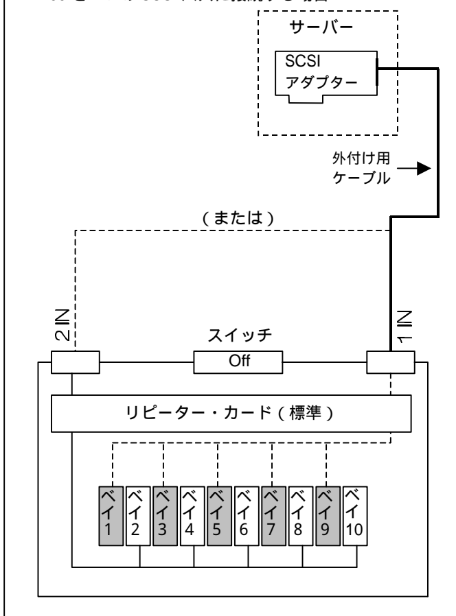
EXP200 を 1 つの SCSI バスに接続する場合
