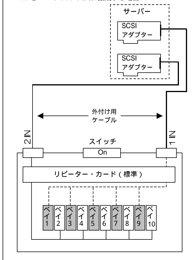
EXP200 を 2 つの SCSI バスに接続する場合
