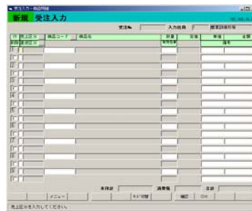
GUI画面
