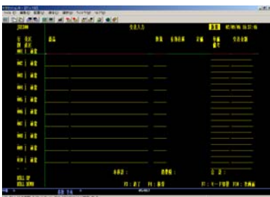
5250画面
