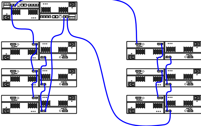
サンプル構成⑤ (DS4700、EXP810 6台以上構成)
