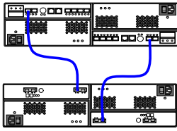
サンプル構成① (DS4700、EXP810 1台構成)
