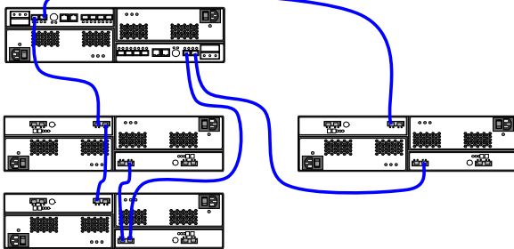
サンプル構成③ (DS4700、EXP810 3台構成)
