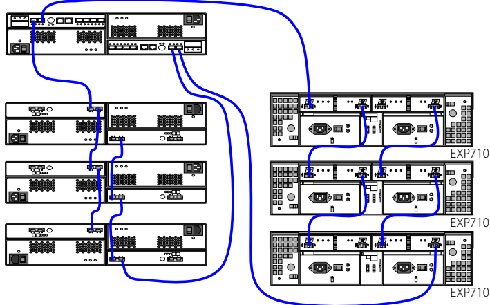
サンプル構成⑥ (DS4700、EXP810とEXP710の混在構成)
