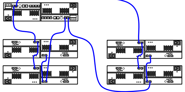
サンプル構成④ (DS4700、EXP810 4台構成)
