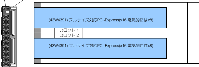
HS21(8853) BladeCenter PCI 拡張ユニット IIもしくはPCI EXPRESS I/O 拡張ユニット
