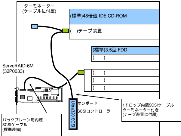
ServeRAIDコントローラーにHDDを接続している場合
