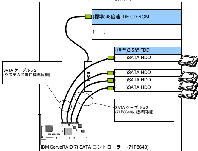
SATA RAID コントローラー構成図
