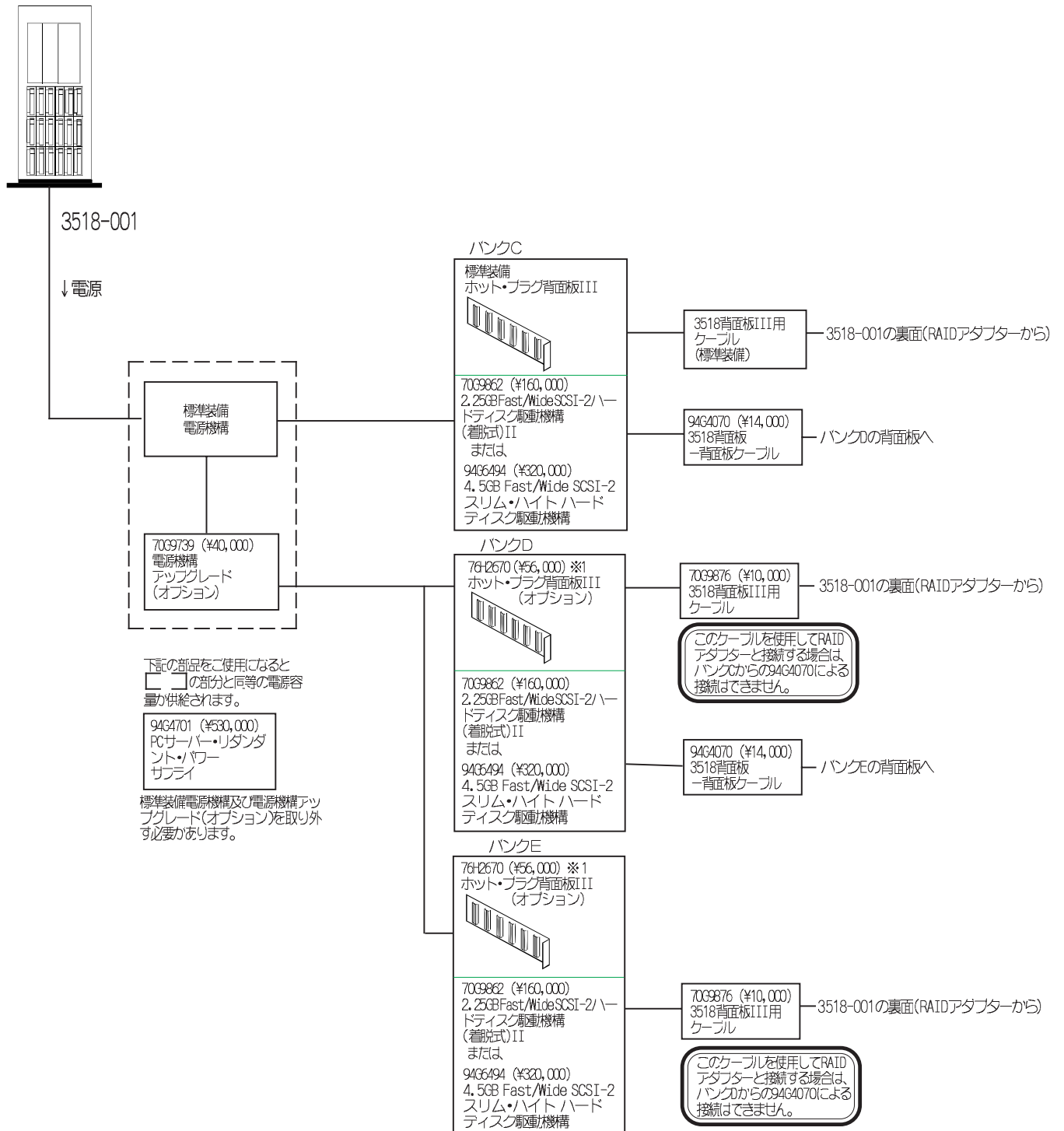
3518 SCSI記憶機構格納装置 接続図
